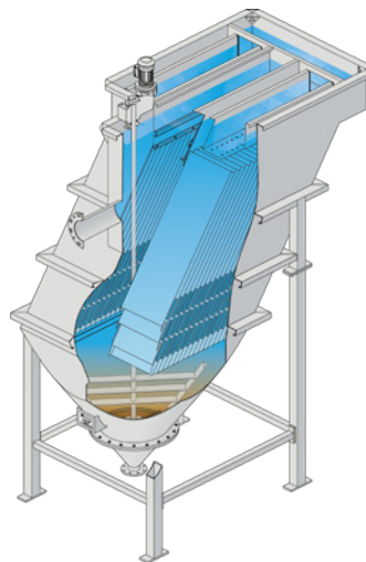
Lamella LS mit Schlammkrählwerk
